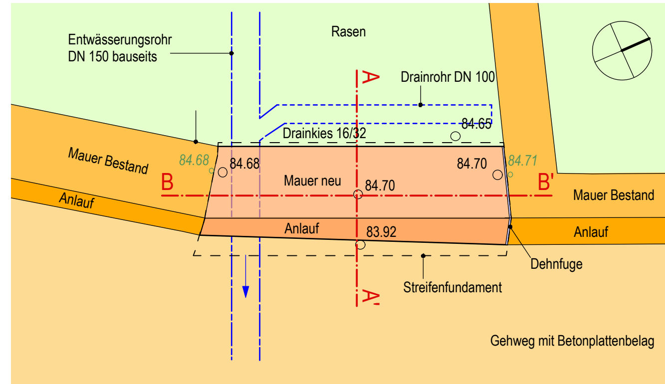
GRUNDRISS
